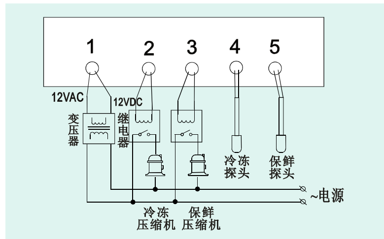
接线图
