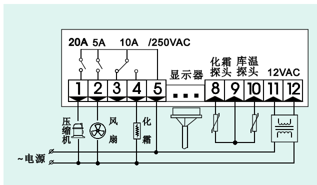
接线图
